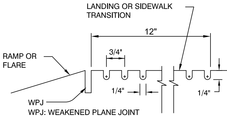
12" GROOVING DETAIL
